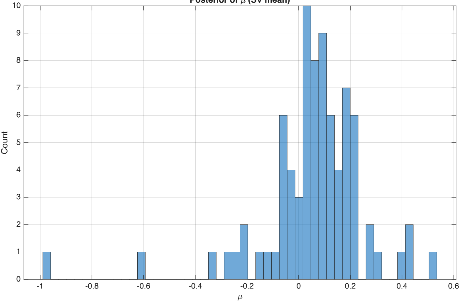
Posterior of \mu (SV mean)
